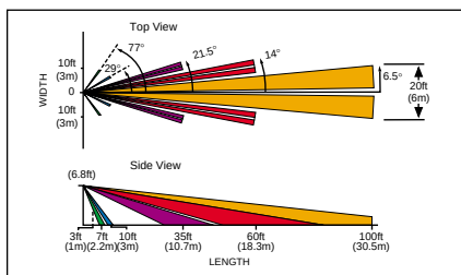
LONG RANGE LENS (P/N D 02)
